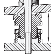
Arandelas de nivelación GN 350.3
