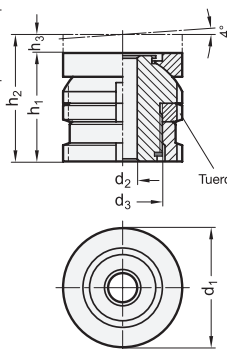
Arandela GN 6339
